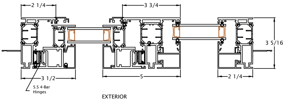
OA Window
